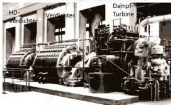
Gas-Turbinenkompressor, Gesamtansicht
