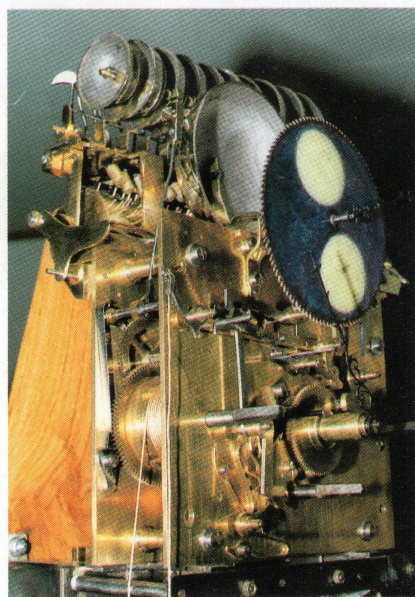
Abb. 4: Unterzifferblattansicht mit der Mondphase
