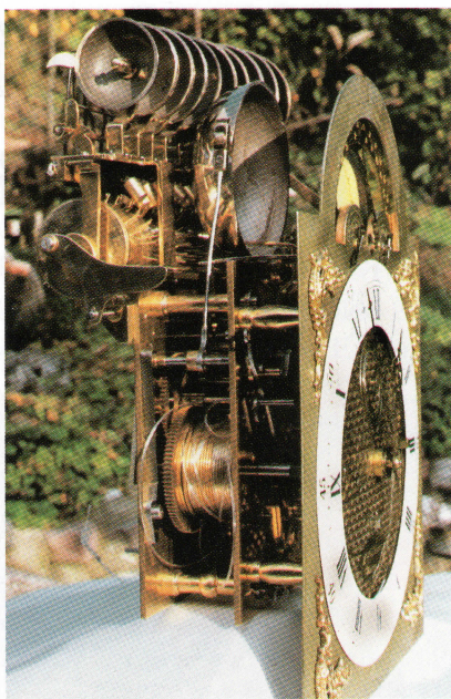
Abb. 3: Seitlicher Blick ins Werk mit der Musikwalze und den 10 Glocken
