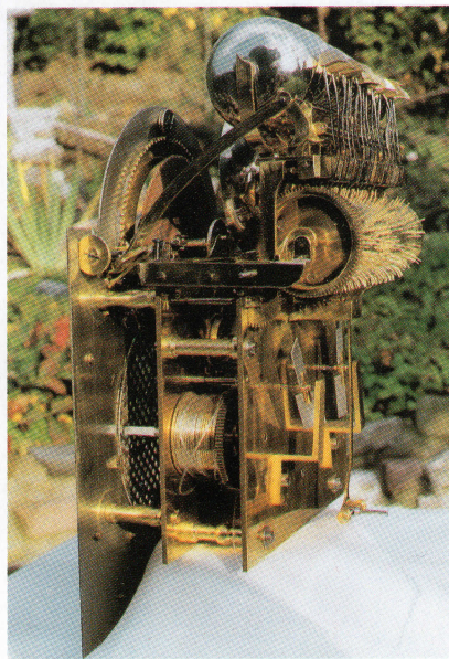
Abb. 5: Werk von hinten mit Walze, Hämmern und zwei Windfängen
