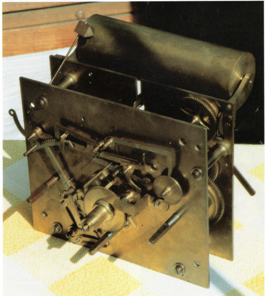
Abb. 1: Das Uhrwerk mit Musikwalze wie es beim Trödler gefunden wurde
